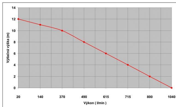
Přenosné plovoucí čerpadlo 800/190
